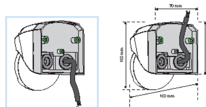
Kableinführung von unten oder von oben
